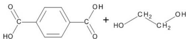
Acide téréphtalique
