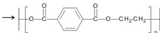
Polyéthylène téréphtalate
