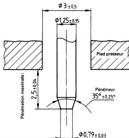
Figure 1 - Pénétrateur pour le duromètre du type A
