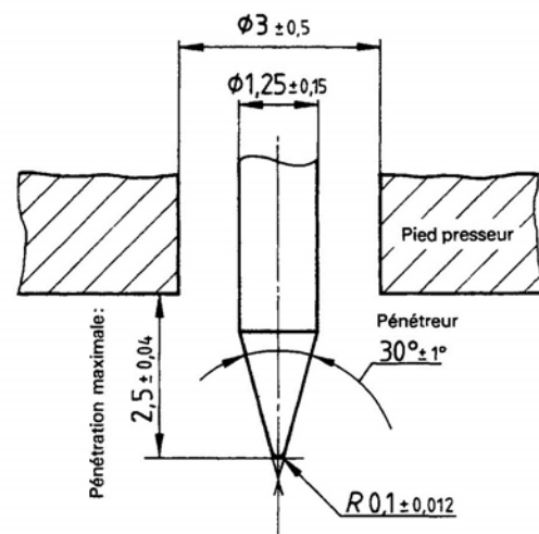
Figure 2 - Pénétrateur pour le duromètre du type D
