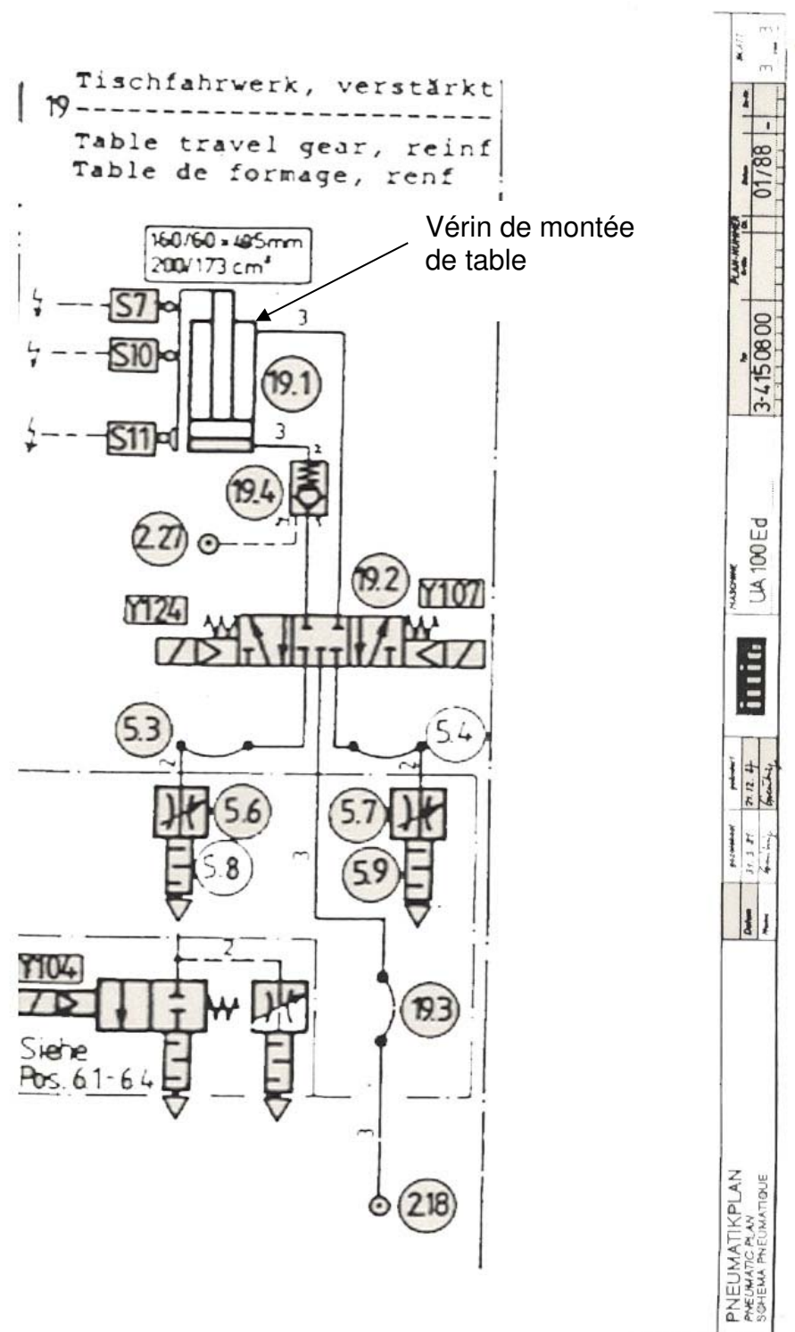
Extrait du schéma pneumatique de la thermoformeuse Illig UA
